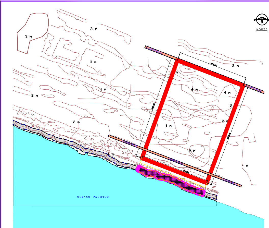
CUADRO DE CONSTRUCCION ZONA FEDERAL MARITIMA
